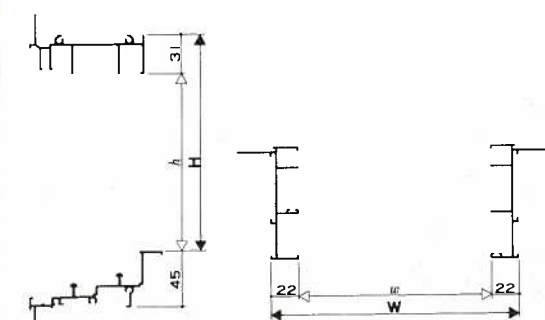
●テラス型
